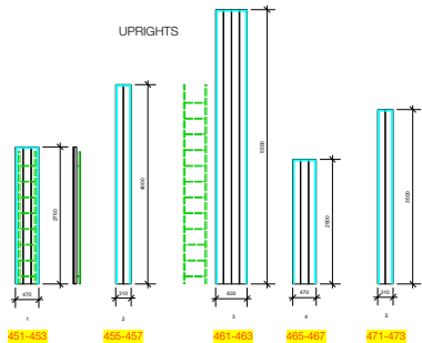
5 Uprights Scale: 1:50
