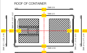
2 Roof Scale: 1:50
